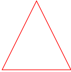
Triángulo isósceles
