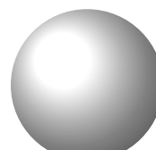
Esfera
