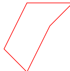
Figura asimétrica
