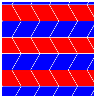
Teselado
