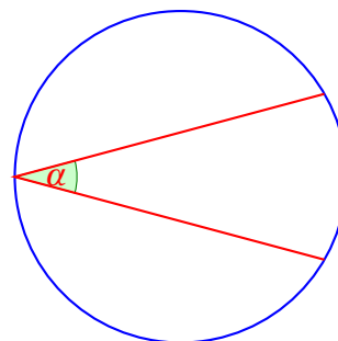
Ángulo inscrito
