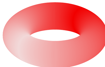
Toro
