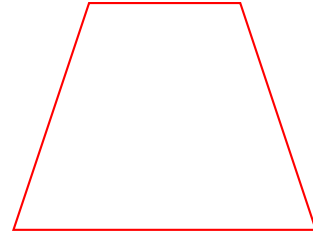
Trapezio isósceles
