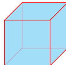
Cubo
